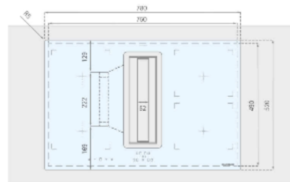
Kochfeld – Aufsatzmontage
