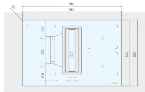
Kochfeld – flächenbündige Montage
